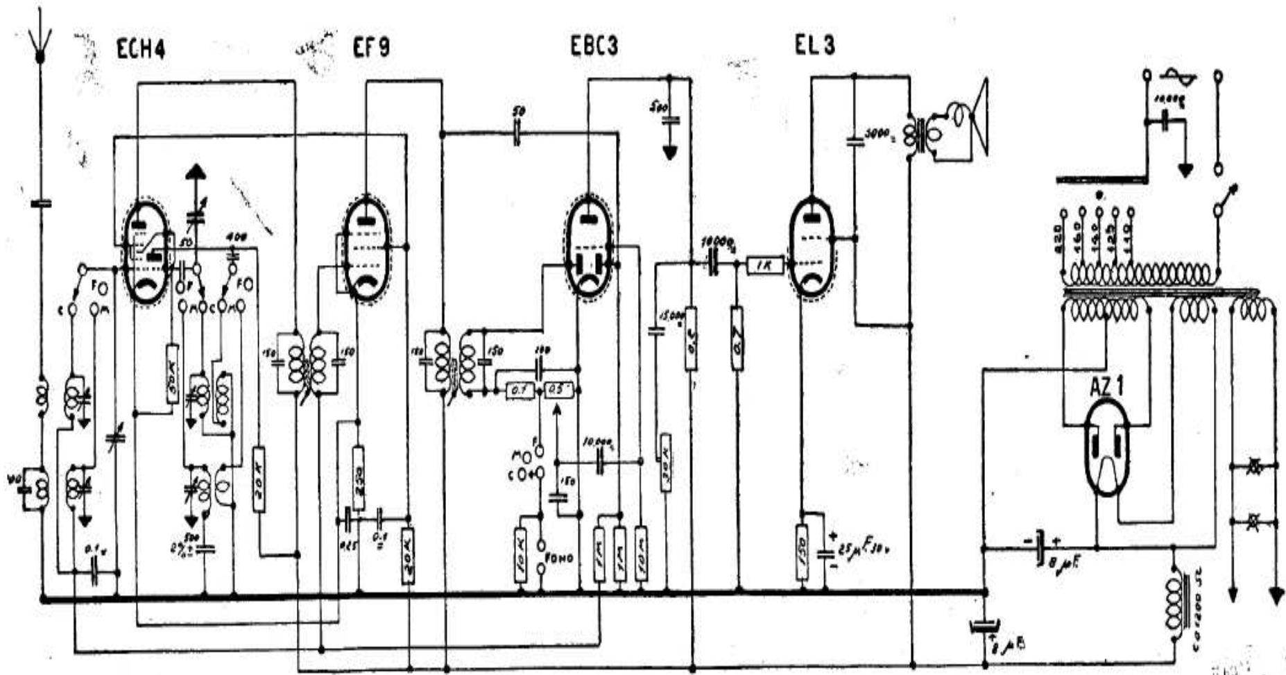
BERTONCINI RADIO - Mod. T 89 - Onde medie e corte. Media frequenza: 468 kc. Bobina campo: 1200 ohm. Potenza d'uscita: 2 watt.
